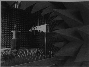
Hérissé de pyramides de mousses absorbantes, la cage de Faraday qui vient d'être installée au CNET de Lannion par la SIEPEL (photo CNET - M. Le Gall).
