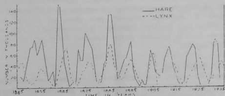
Fig. 4. Oscillations des populations de lièvres et de lynx au Canada
