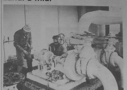
A l'issue des eaux de Kergomar qui a été inondée, on remet les moteurs en place. Ils avaient été démontés dimanche matin. L'usine a pu fonctionner dès le lundi soir (lundi à midi).
