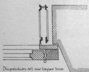
Disposition n°1 sur tapée bois
