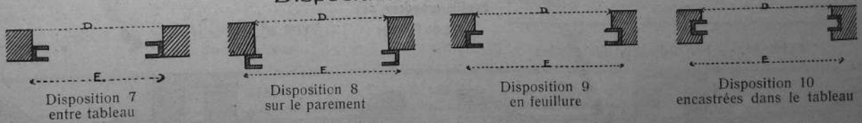
Enroulements intérieurs
