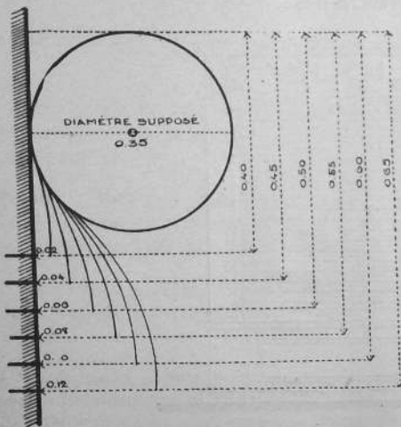
Profil des Ondulations
