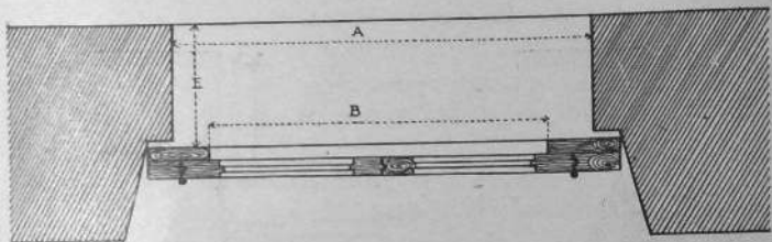
Coupe Horizontale de la Baie
