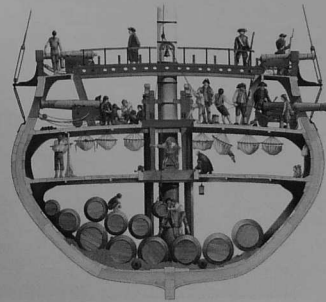
← La frégate, coupe transversale au niveau du maître bau.
